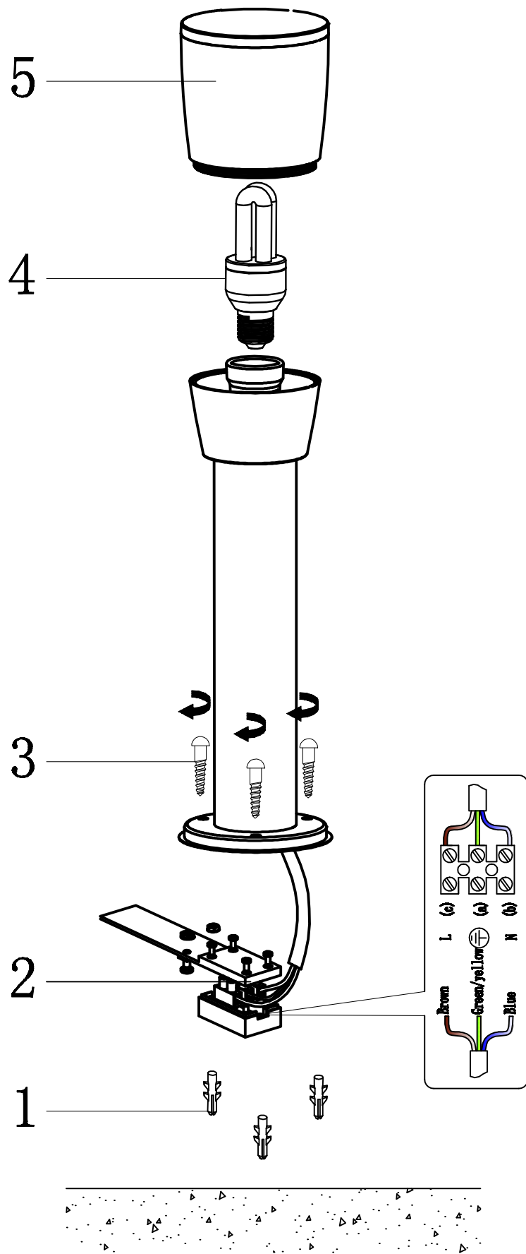
C0587H 安装图
